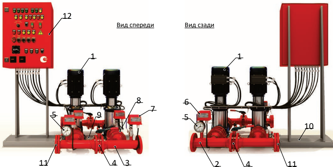
Рисунок 4. Спецификация насосной установки АкваСЕТ П дренажного типа.
