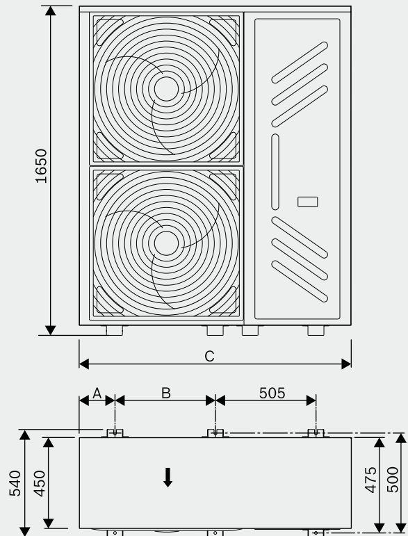
Размеры (в мм) блоков серии MDCI мощностью 40–45 кВт
